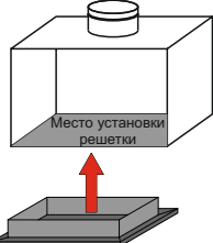
Прямая врезка (ПВ)
