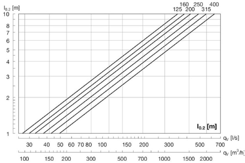
Коррекция длины струи l_{0.2}
